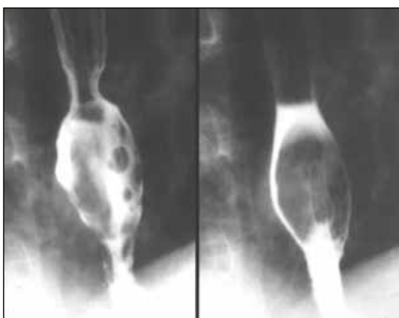
U Abrikosoff
