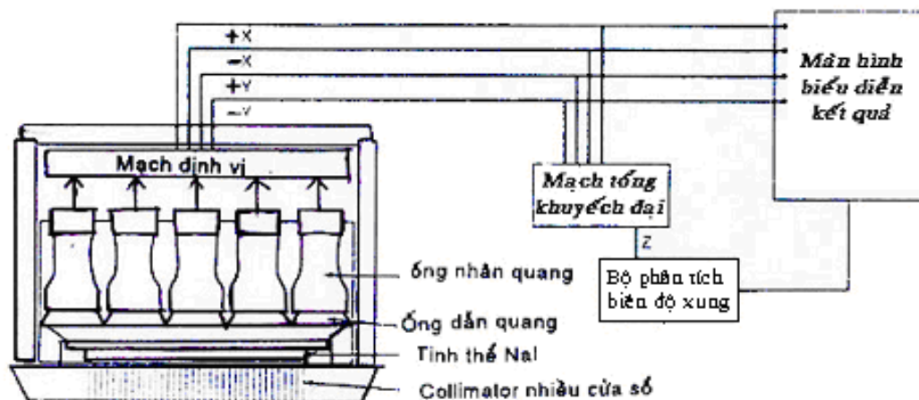
Hình 2.5: Sơ đồ khối của Camera nhấp nháy Anger cho thấy những phần chính của hệ thống ghi hình.
