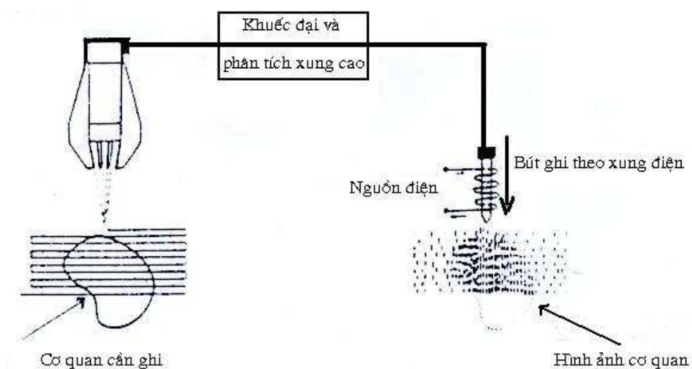
Hình 2.4: Máy xạ hình vạch thẳng (Rectilinear Scanner) với Collimator hội tụ và bộ bút ghi theo tín hiệu xung điện tỷ lệ với hoạt độ phóng xạ trên cơ quan cần ghi, kích thước hình theo tỷ lệ 1:1.
