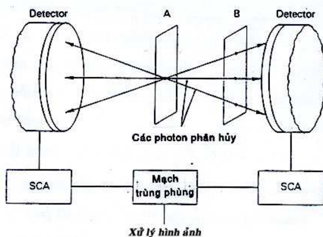
Hình 2.7: Sơ đồ ghi hình Positron bằng cặp đầu đếm trùng phù với các tia \gamma 511 keV.
