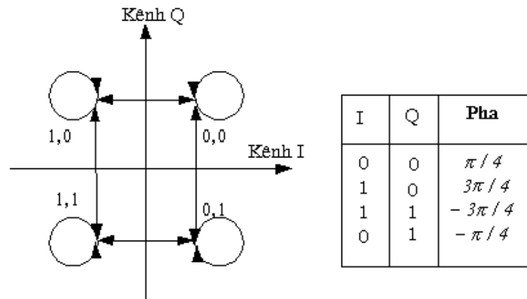
Hình 4.20. Trãi phổ trực giao kênh CDMA hướng lên CDMA được đối chiếu với điều chế QPSK bù như hình 4.20
