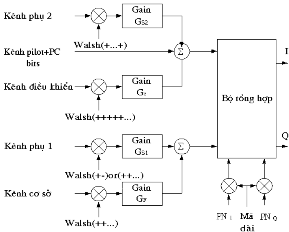
Hình 3.19. Cấu trúc kênh hướng lên
