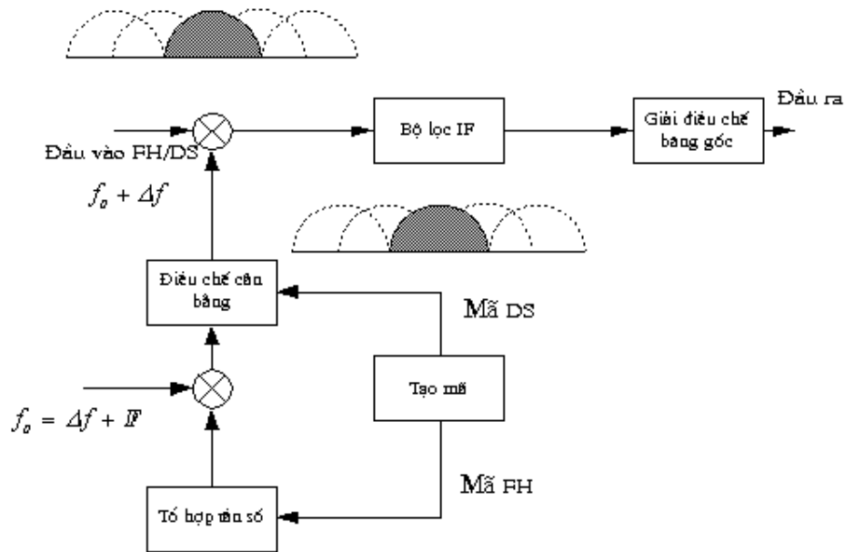
Hình 2.14. Bộ thu tổng hợp FH/DS
