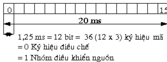
Hình 4.19. Khung kênh CDMA hướng lên
