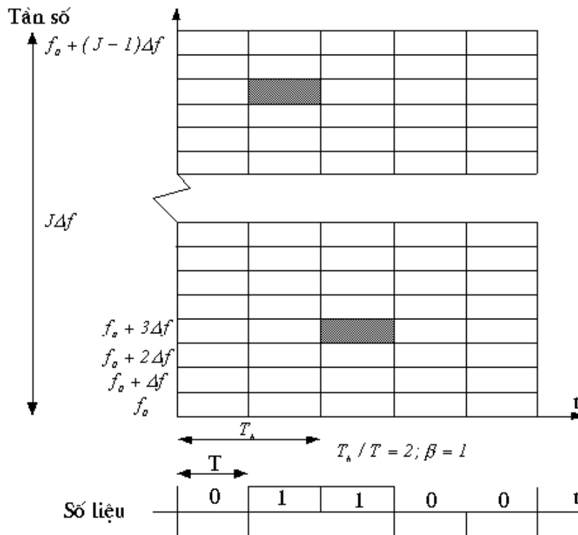
Hình 2.9. Biểu đồ tần số cho một hệ thống FH chậm điều chế FSK cơ sở hạ
