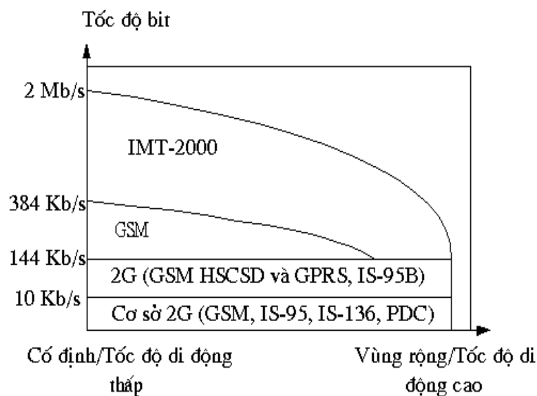
Hình 3.4. IMT-2000
