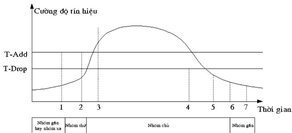
Hình 4.16. Quá trình chuyển rập khi thay đổi ngưỡng
