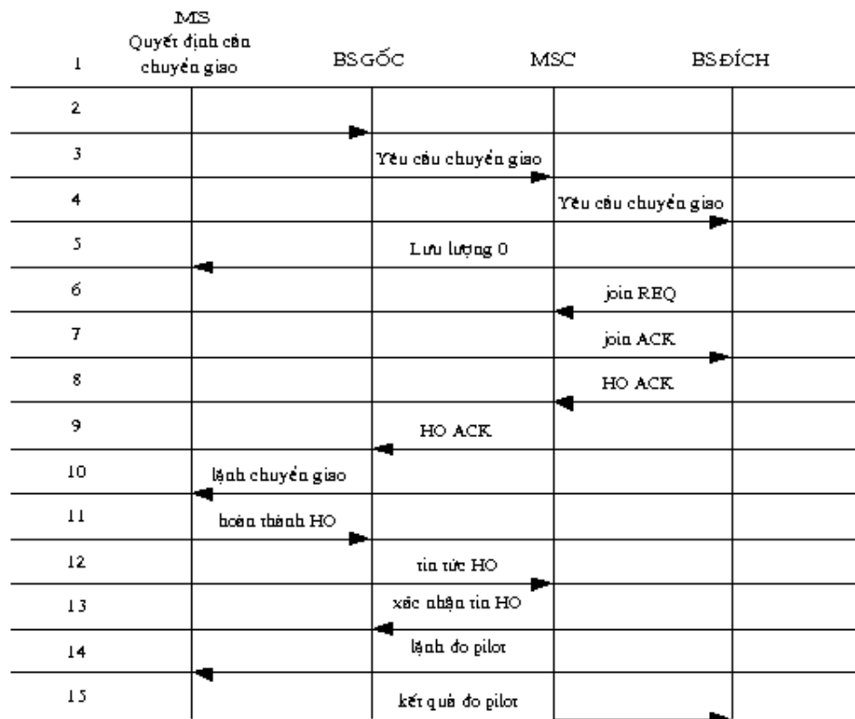
Hình 4.10 . Bắt đầu quá trình một chuyển giao mềm
