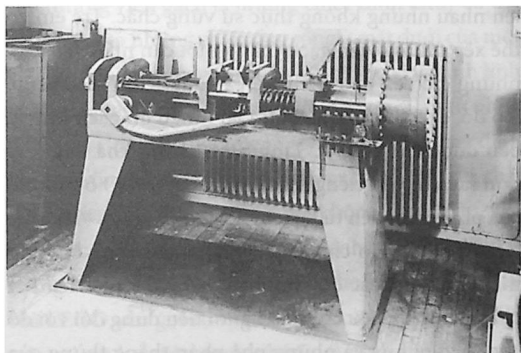
Một chiếc máy ép phun nhựa của LEGO vào năm 1947.
