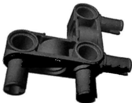
Chi tiết “Hassepin” được thực hiện dựa trên ý tưởng của Steve Hassenplug: một linh kiện giúp hai thanh dầm Technic có thể gắn đúng góc với nhau.
