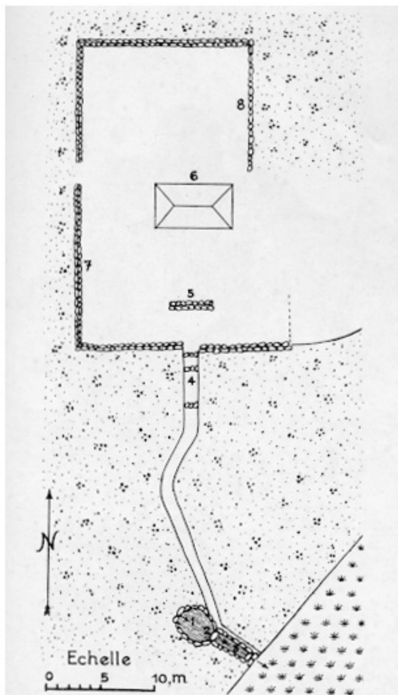
Planche LXXXVIII. — Bassins Quàn (village de Gia-Binh). — Plan : 1, bassin d'alimentation. 2, pont. 3, chenal d'écoulement. 4, entrée de l'enceinte. 5, mur écran protégeant l'entrée de la maison commune, peut-être postérieur aux autres murs. 6, maison commune. 7, murs épais, hauts de 1m.15. 8, rangée de pierres basses.
