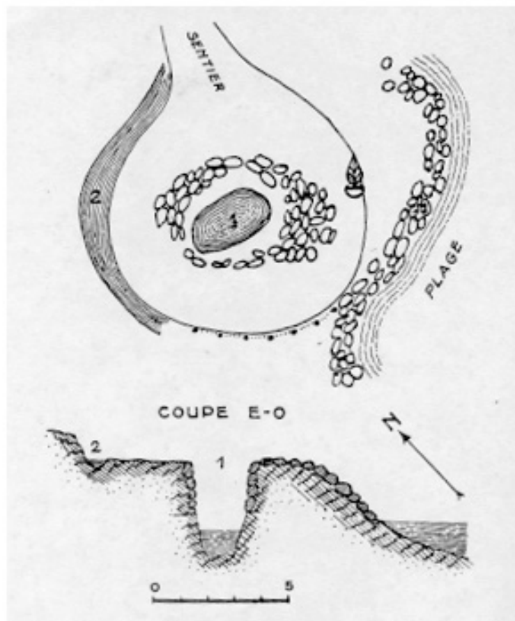
Planche CXCI. — Ce puits ne porte aucun nom. Village de Thuỷ -Cần. Hameau Vinh. Coupe et plan : 1, puits. 2, fossé dans lequel s'écoule à l'occasion l'eau gaspillée par les porteurs. Au Sud -Sud -Est, la plage et la mer. .
