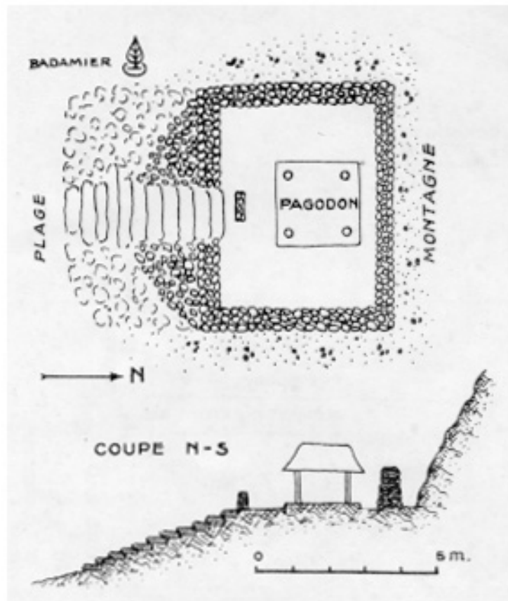
Planche CXCH. — Pagodon du Génie de la mer. Village de Thủy-Cần. hameau de Vĩnh. Coupe dessinée sans mesures. Plan. L'escalier mène à la plage.
