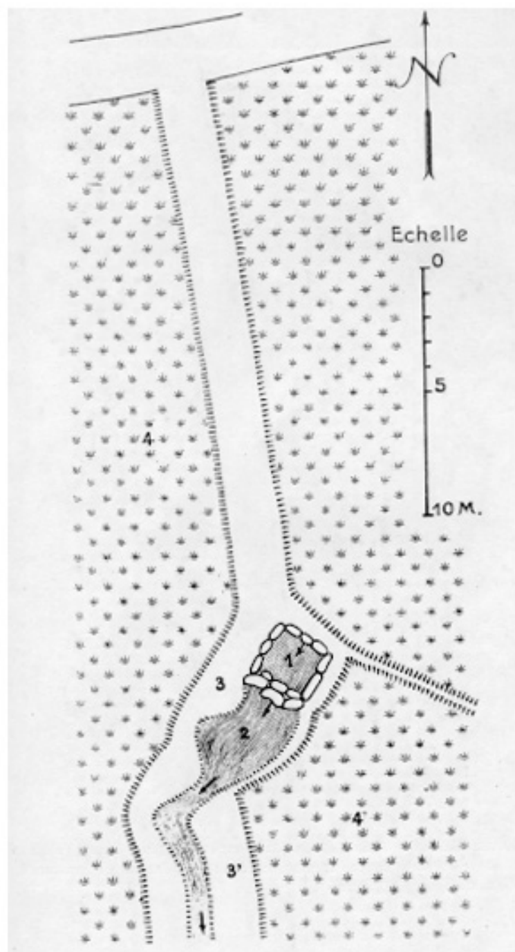
Planche CLXX. — Puits Đường Bát. Village de Hồ-Xá — Plan :
