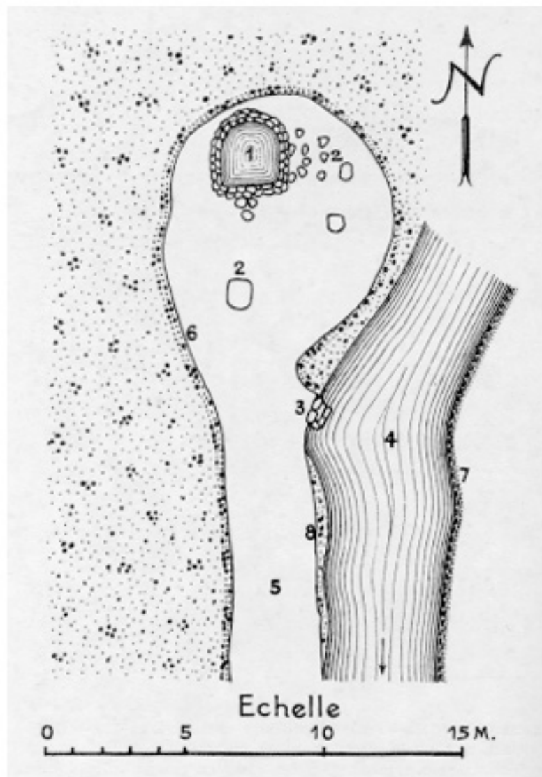
Planche CLXXIX. — Puits Sóng, Village de Liêm - Công - Tây — Plan : 1, puits ; profondeur totale 2m. 56 (de l'eau 88cm). 2, pierres plates. 3, escalier permettant aux laveuses de descendre. 4, cours d'eau (courant rapide). 5, route. 6, haie. 7, rive escarpée du cours d'eau. 8, bord ; hauteur au -dessus de la surface de l'eau : 1m. 24.
