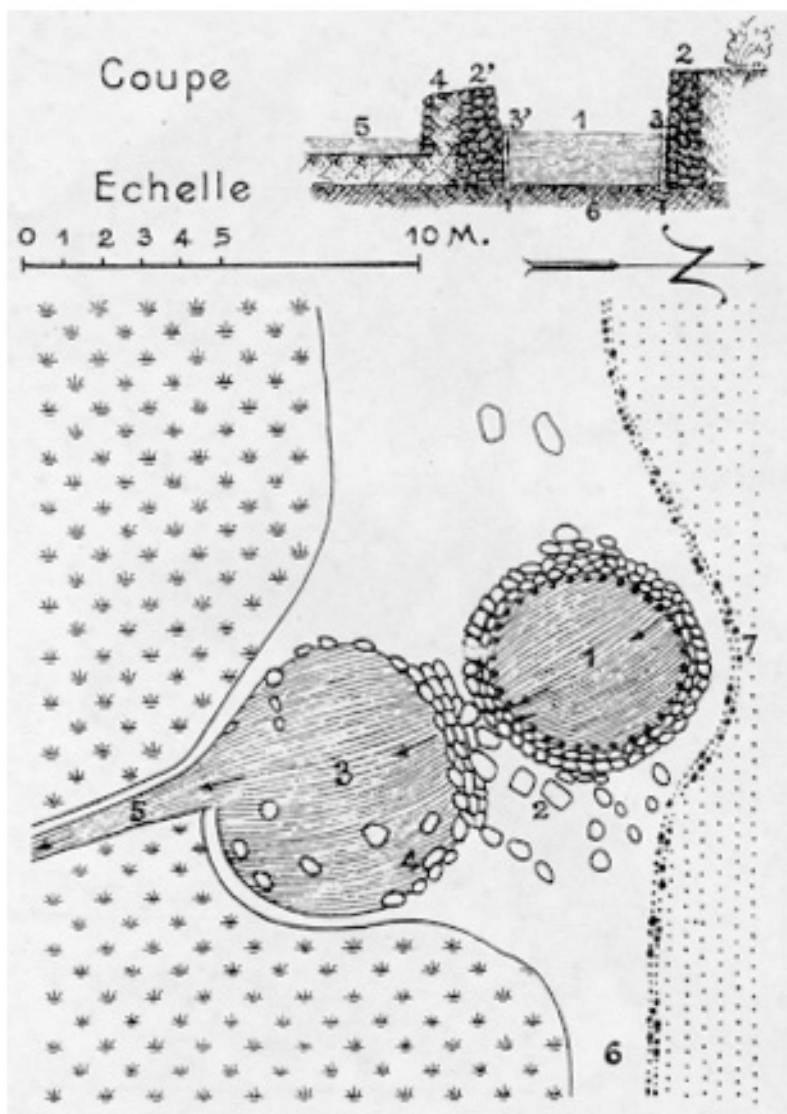
Planche CLXXIII. — Puits Dan. Village de Liêm -Công -Đông — Coupe : 1, puits. 2, 2', parois en pierres naturelles, non maçonnées.
