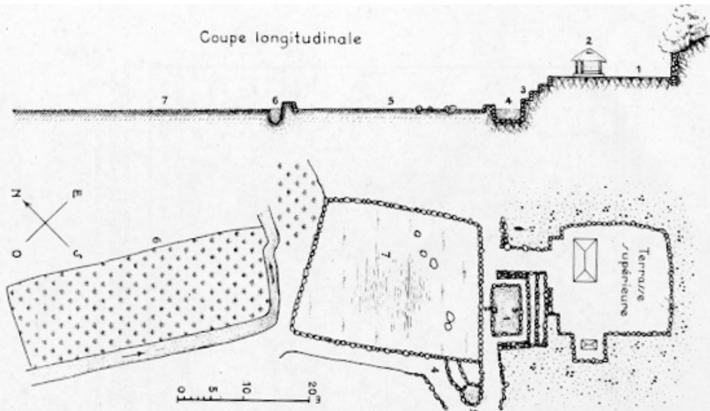
Planche LXXXV. — Bassin Bung ( village d'An -Nha ) — Plan : 1, bassin d'alimentation. 2, escaliers du bassin. 3, mur. 4, route plate. 5, petit bassin. 6, rizières. 7, grand bassin. Coupe : 1, terrasse supérieure. 2, Dinh. 3, mur 4, bassin d'alimentation. 5, grand bassin marécageux. 6, petit cours d'eau. 7, rizières. ( Voir Pl. X.)
