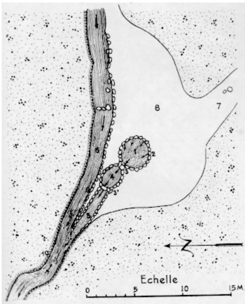
Planche CLXXII. — Puits Mũ Trũm. Village de Liẽm -Công -Đông — Plan : 1, puits, eau potable. 2, mur. 3 et 3', ponts. 4, bassin où l'on lave le linge. 5, chenal d'écoulement confluant avec le cours d'eau 6 et 7, route très en pente menant au haut du plateau. 8, aire presque plate. 9, digue construite mesurant près d'un mètre au -dessus de l'eau. 10, talus.
