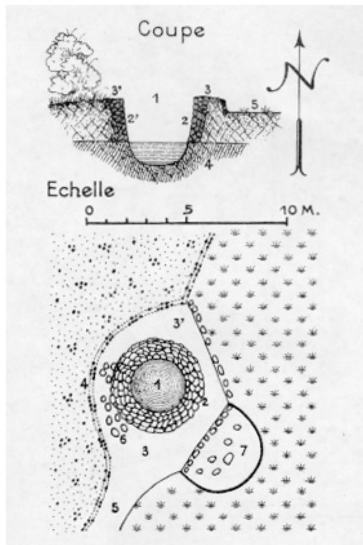
Planche CLXXIV. — Puits Rô. Village de Liêm -Công -Đông — Coupe : 1, puits. 2, 2', parois. 3, 3' plates -formes. 4, rocher (basalte). 5, rizière plate.
