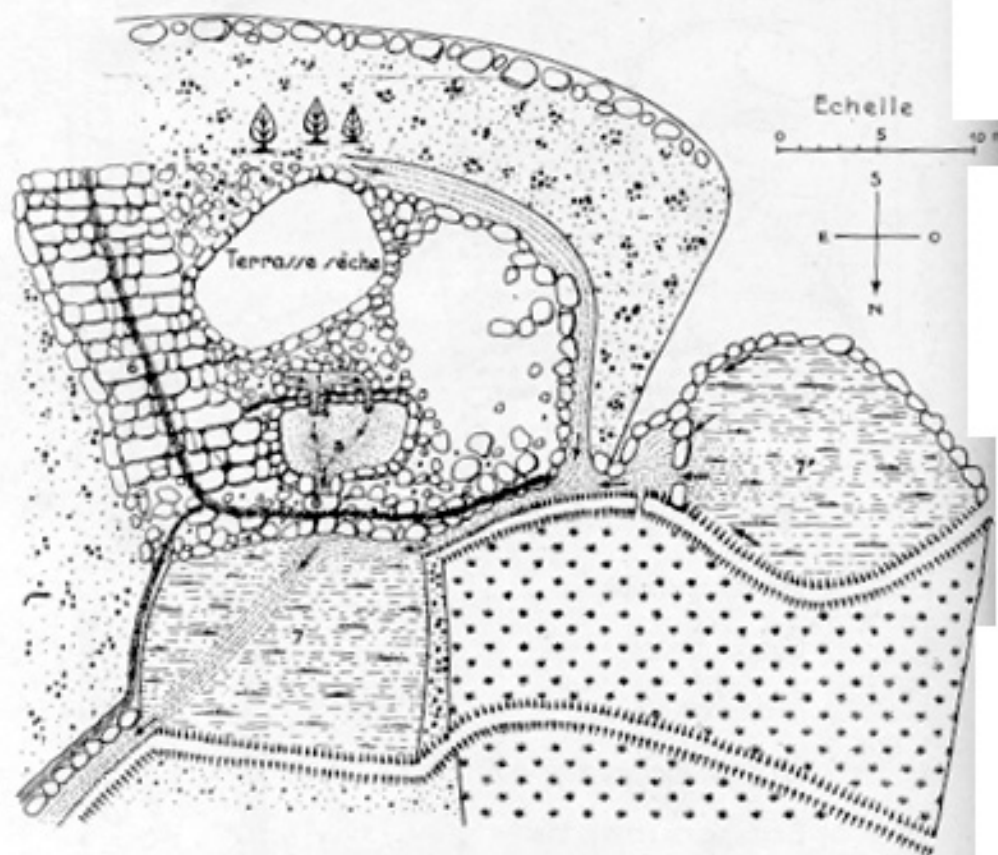
Planche LXXI. — Bassin Đào ( village d'An -Nha ). — Plan : 1, petit bassin. 2, mur. 3, terrasse sèche. 4, bec de cuve. 5, bassin d'alimentation. 6, escalier. 7, grand marécage. 8, pont. ( Voir Pl. XVI à XX. )
