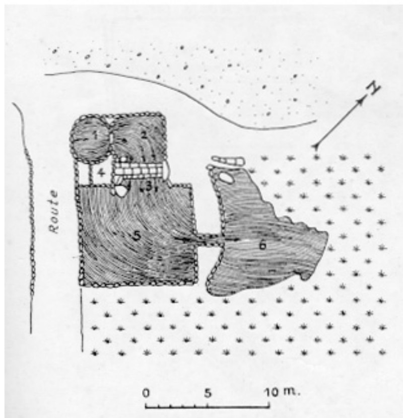
Planche XCVI. — Bassin Sâu (village de Xuân-Hòa) — Plan : 1, bassin de réception. 2, bassin d'alimentation. 3, pierres équarries, peut-être récentes. 4, sorte de petit terrasse. 5, bassin de lavage. 6, bassin presque stagnant.
