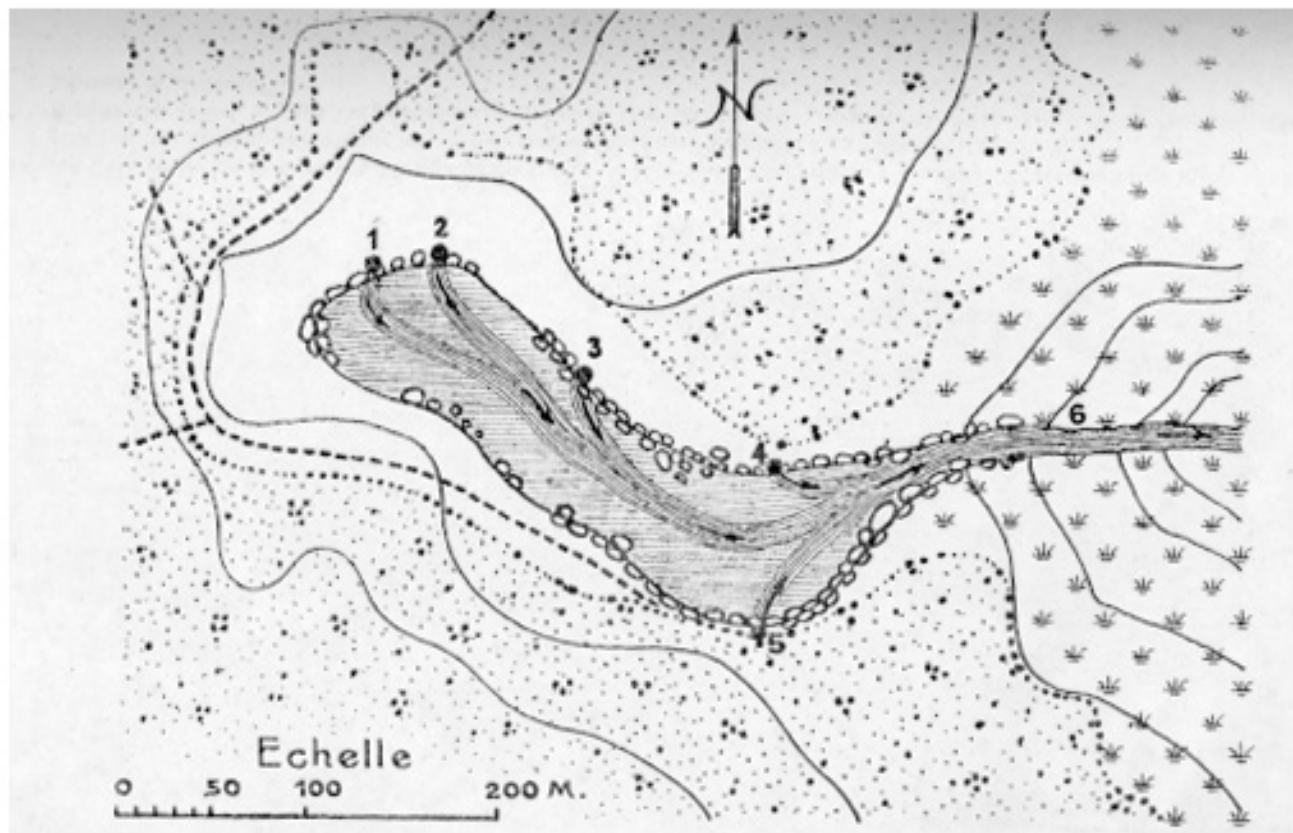
Planche CII. — Khe Cù (village de Hào-Sơn), déversoir de cinq bassins — 1, bassin Bà (Madame). 3, bassin Voi (Eléphant). 4, bassin Gái (Fille). 5, bassin Diêm. 6, défluent coulant vers les terres basses. 2, bassin Ông (Monsieur). Courbes de niveau de 5 en 5 m. (Voir Pl. VI).
