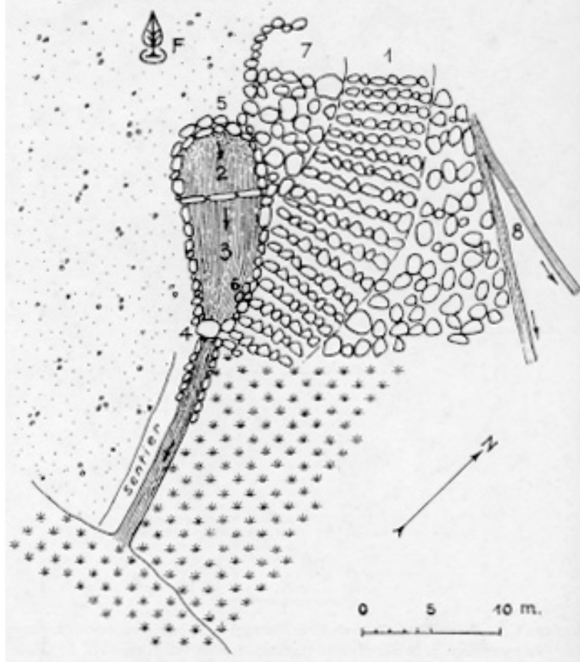
Planche CI. — Bassin Da (village de Nam -Tây) — 1, escalier en pierres brutes, mène au haut de la côte. 2, bassin de réception. 3, bassin d'alimentation. 4, pont fait d'une seule pierre. 5, mur élevé. 6, petit escalier du bassin. 7, ancienne terrasse ou bassin. 8, deux ruisseaux divergents coulant dans les pierres.
