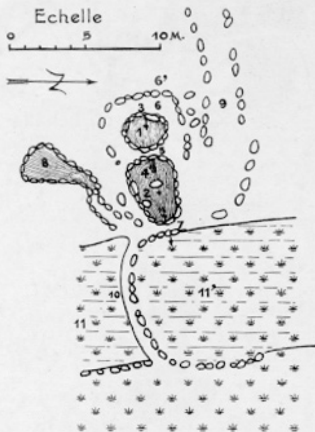
Planche LXXXIII. — Bassin Môt ( unique ) ( village de Long - Son ) — Plan : 1, bassin supérieur. 2, bassin d'alimentation. 3, mur. 4, bec de cuve en bois ( distance entre le bec de cuve et la surface de l'eau 95 cm.). 5, pont. 6, terrasse supérieur sèche. 6', grande terrasse. 7, pont Est. 8, bassin d'eau stagnante. 9, route. 10, diguette. 11, et 11', rizières en terrain plat, inondées.
