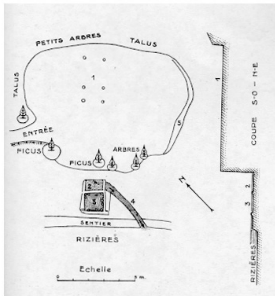
Planche CLXXVI. — Bassin Hố (Hố = escalier). Village de Hoàng Công — Coupe dessinée sans mesures ; les hauteurs sont exagérées. Plan et coupe : 1, sur la terrasse, emplacements des poteaux pour le pagodon éphémère des cérémonies. 2, eau provenant du talus. 5, eau presque stagnante ; l'armature des bassins 2 et 3 est en bois. 4, défluent. 5, remblai en terre.
