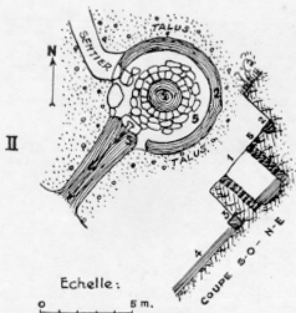
Planche CLXVIII, I. — Puits Thiêt, Village de Đon -Duệ. Plan et coupe :
