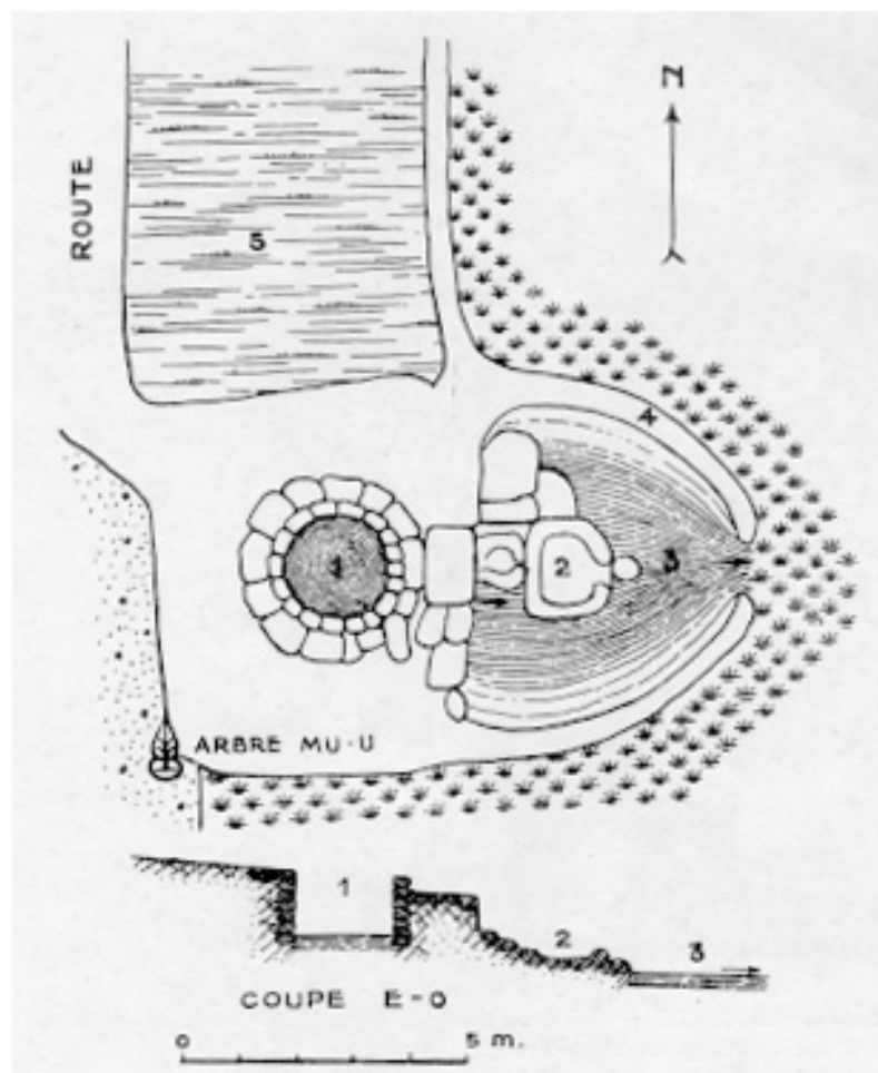
Planche CLXXXVIII. — Deuxième puits Mù -u. Village de Thuý -Trung.
