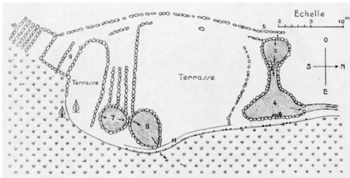
Planche XCI. — Bassin Dia ( village de Gia-Binh) — Plan : 1, mur (haut de 1m.87). 2, bassin supérieur. 3, pont. 4, bassin presque stagnant. 5, terrasse. 6, escalier permettant de descendre dans le bassin. 7, 8, deux bassins communicant, eau presque stagnante. 9, route. 10, escalier bas. 11, sentier bordé d'une haie. (Voir Pl. VIII, à droite.)
