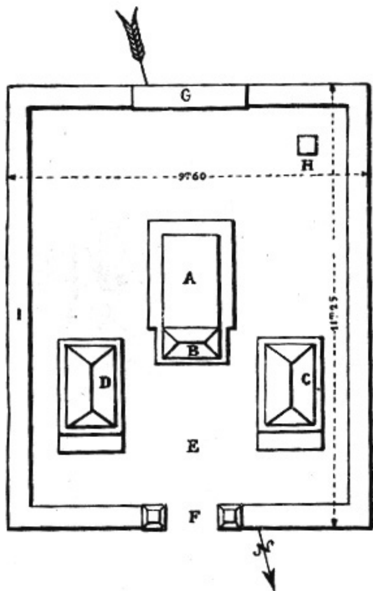
Planche CXIX. — Tombeau N° 307 : plan ( Dessin de M. Nguyễn - Thứ ).
