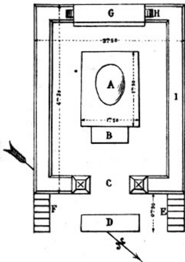
Planche LXIX. — Tombeau N° 202 : plan ( Dessin de M. Nguyễn - Thứ ).
