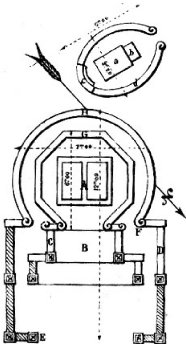
Planche CXIV. — Tombeau N° 300 -301 : plan ( Dessin de M.Nguyễn -Thứ )
