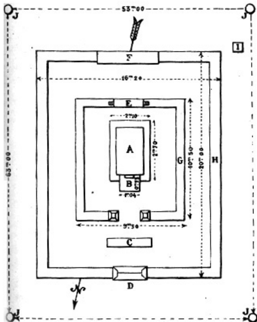
Planche LXXXI. — Tombeau N° 243 : plan ( Dessin de M. Nguyễn -Thứ ).
