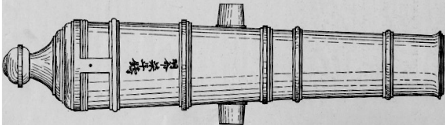
Planche LIII. — Les canons du fortin du Col des Nuages. Echelle : 10 cm. pour 1m. Dessin de M. H. Cosserat, fils.
