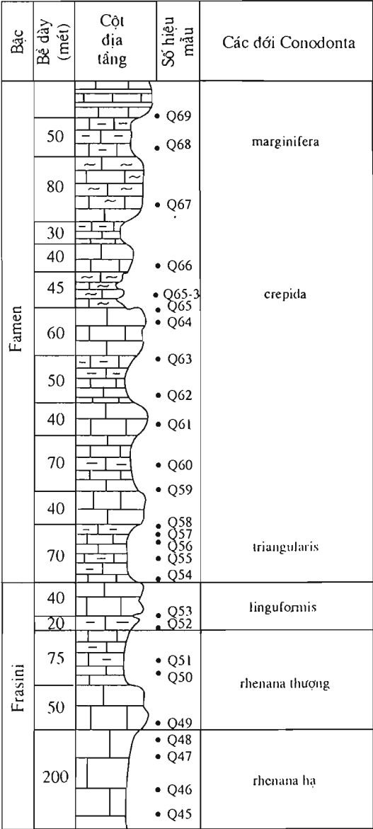
Hình 2.7. Cột địa tầng của khoảng ranh giới F/I 2 ở mặt cắt Xóm Nha
