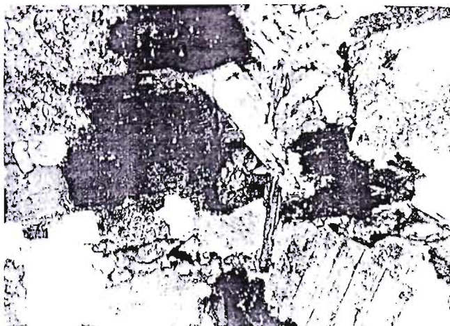
Hình 2.46. Granit hai mica sáng màu, hạt lớn tha hình, plagiocla bị xerixit hoá khối Đồng Hới N + , x40 (ảnh Trần Nghi, Trần Trọng Hoà, 2000)
