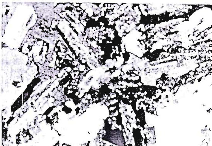
Hình 2.48. Granit hạt trung, kiến trúc nửa tự hình và tự hình Thạch anh tha hình, Plagiocla tự hình và nửa tự hình khối Đồng Hới N + , x40 (ảnh Trần Nghi, Trần Trọng Hoà, 2000)
