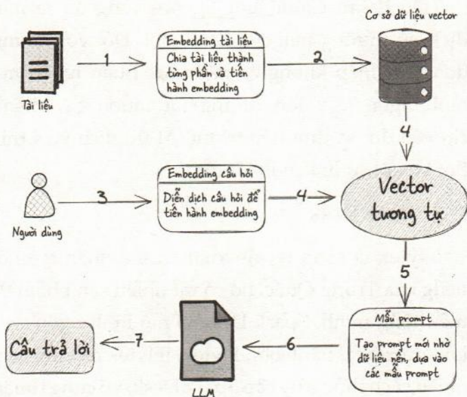
Hình 9-3: Minh họa quy trình chuyển cơ sở dữ liệu vector làm cơ sở tri thức
